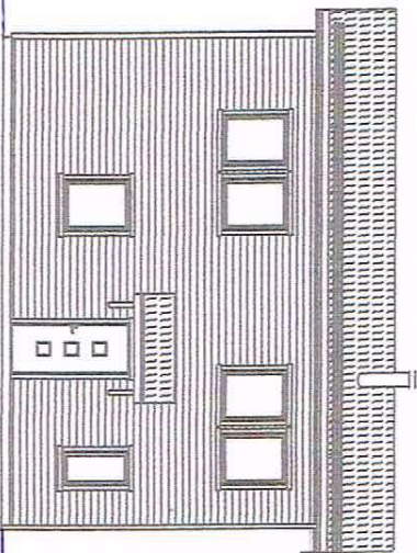
Fasade mot øst Total lengde 9065 mm
