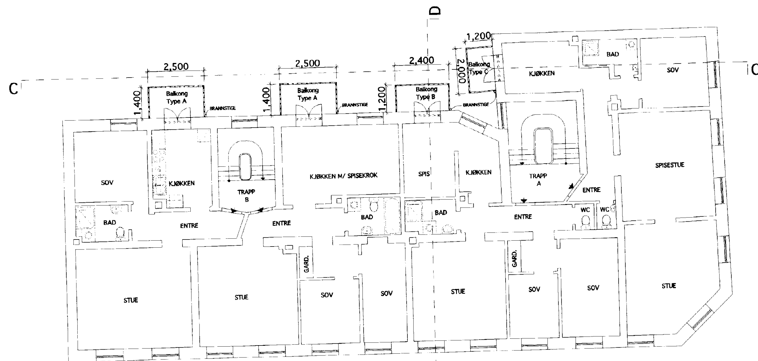
Plan 4. etasje
