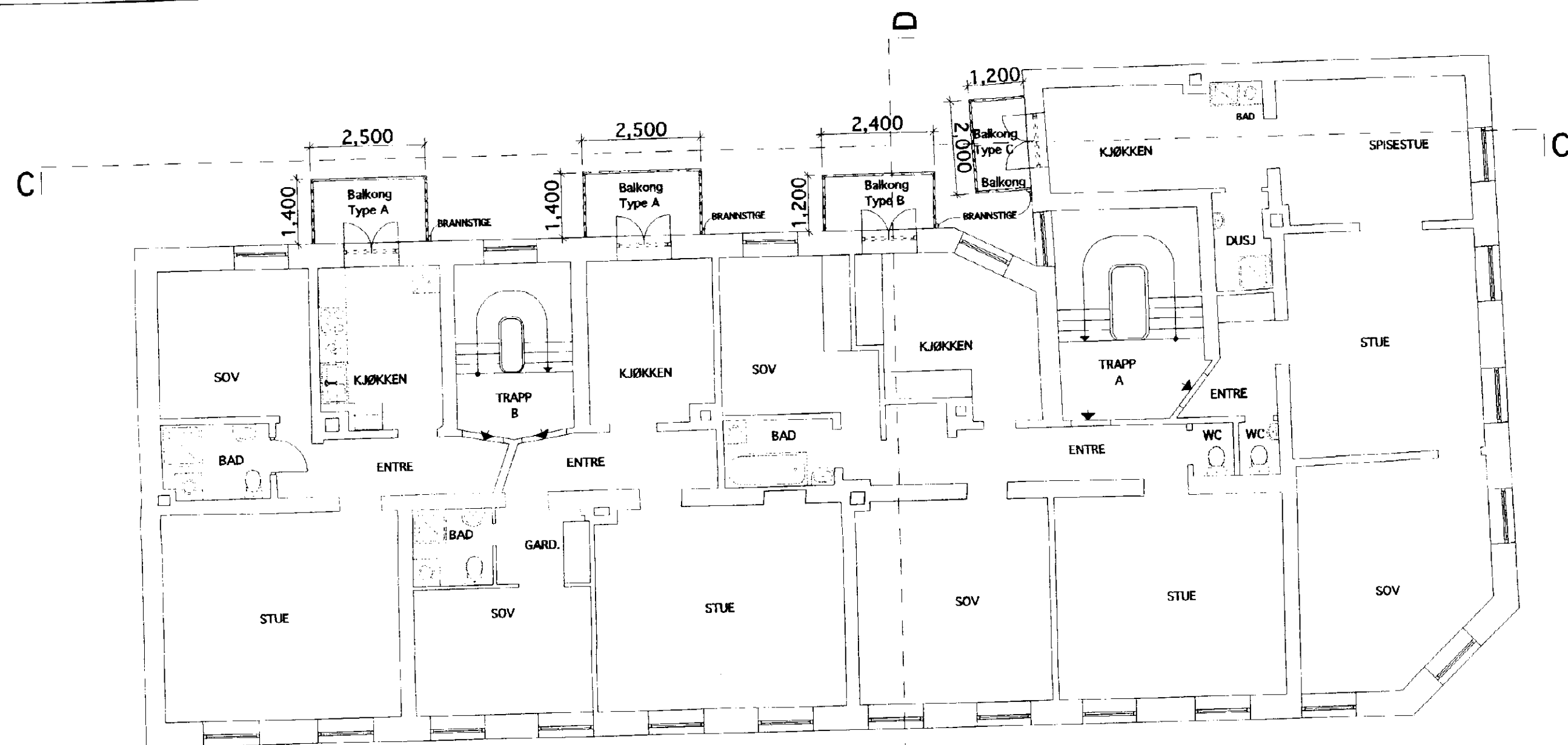
Plan 3. etasje
